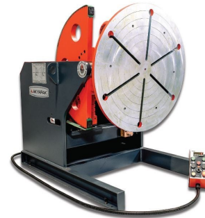
SRP - CONVENTIONAL POSITIONERS AYARLI KAYNAK POZİSYONERİ
